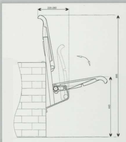
sposób mocowania do ściany
